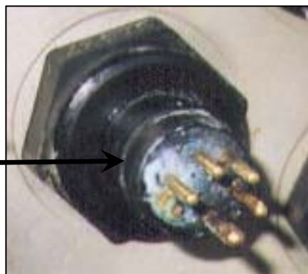
腐食してピンの折れた バルクヘッドコネクター
