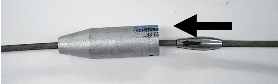
写真c：矢印の方向へ（割れ目のある位置に注意）
