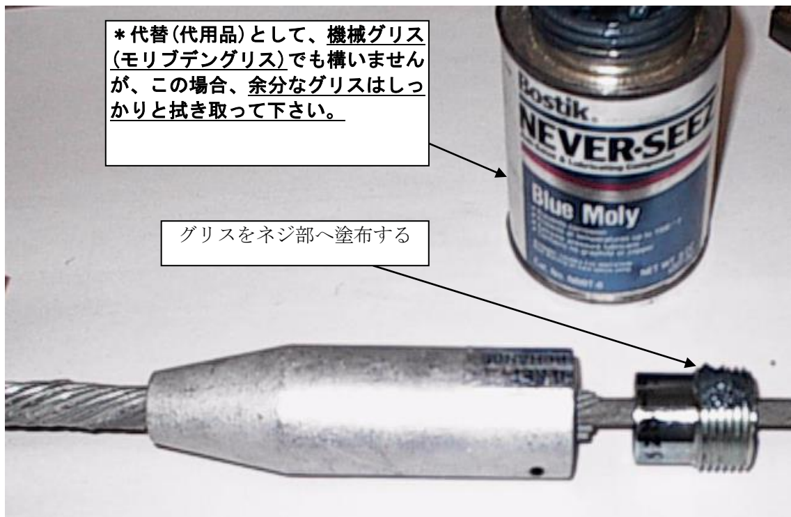
写真h：ネジ部には腐食防止用グリスを塗ること
