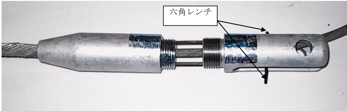
写真 i : 六角レンチは所定の穴へ通します
