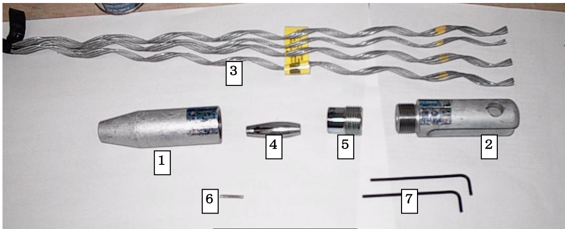
写真 a : パーツ類
