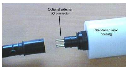
参考写真② : 外部 I/O コネクタ
